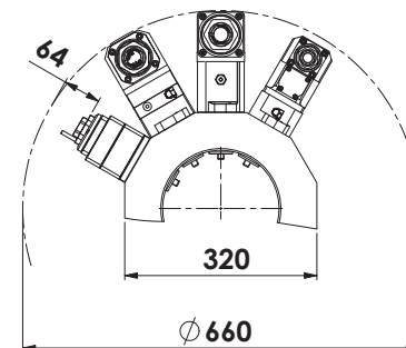
MANDRINO SECONDARIO SECONDARY SPINDLE CABEZAL SECUNDARIO GEGENSPINDEL 第2主軸 ДОПОЛНИТЕЛЬНЫЙ ШПИНДЕЛЬ
