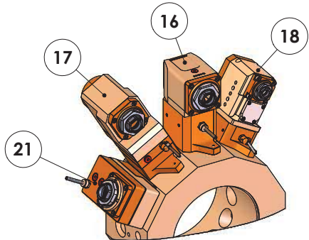
MANDRINO SECONDARIO SECONDARY SPINDLE CABEZAL SECUNDARIO GEGENSPINDEL 第2主軸 ДОПОЛНИТЕЛЬНЫЙ ШПИНДЕЛЬ
