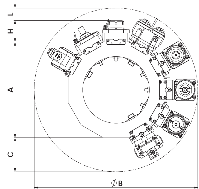
MANDRINO PRINCIPALE E SECONDARIO MAIN AND SECONDARY SPINDLE CABEZAL PRINCIPAL Y SECUNDARIO HAUPTSPINDEL / GEGENSPINDEL 主軸および第2の軸 Главный и дополнительный ШПИНДЕЛЬ
