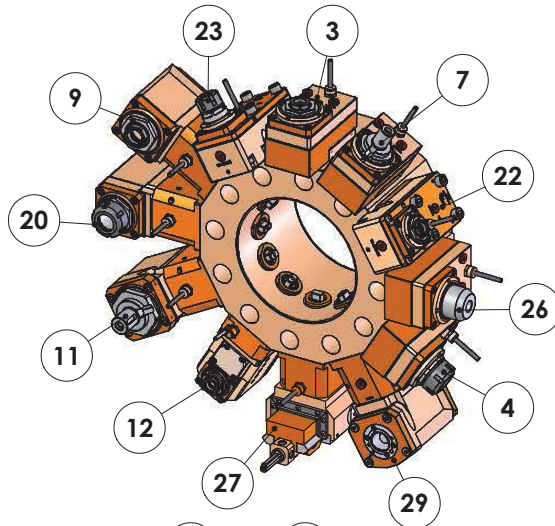
MANDRINO PRINCIPALE MAIN SPINDLE CABEZAL PRINCIPAL HAUPTSPINDEL 主軸 ГЛАВНЫЙ ШПИНДЕЛЬ
