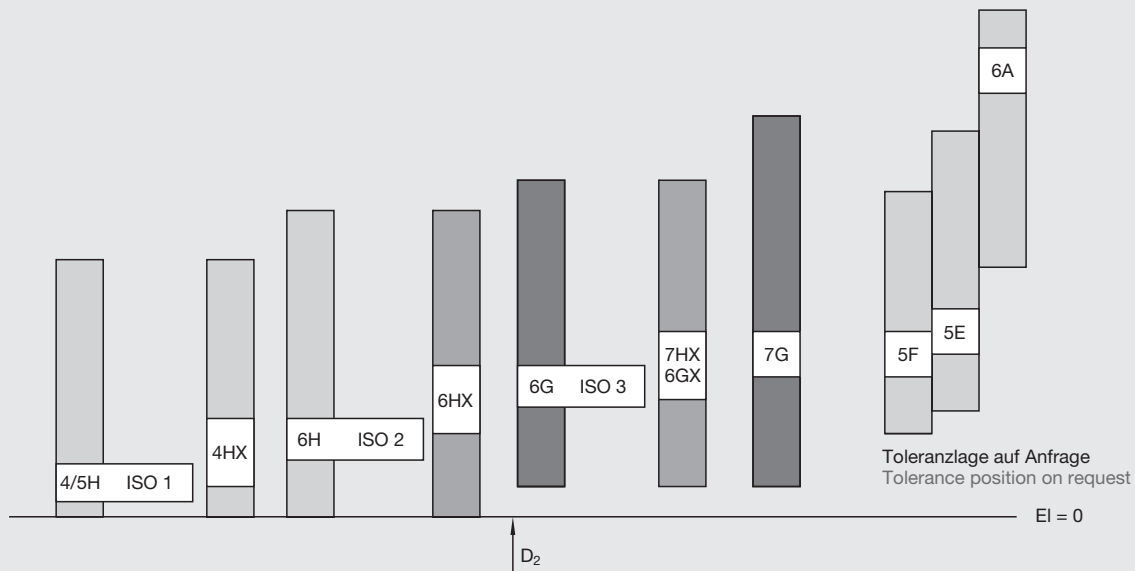
Toleranzlage/-klasse Tolerance position/class
