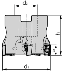
Aufsteckfräser 90° / LNMX ... Face milling cutter 90°/ LNMX ...
