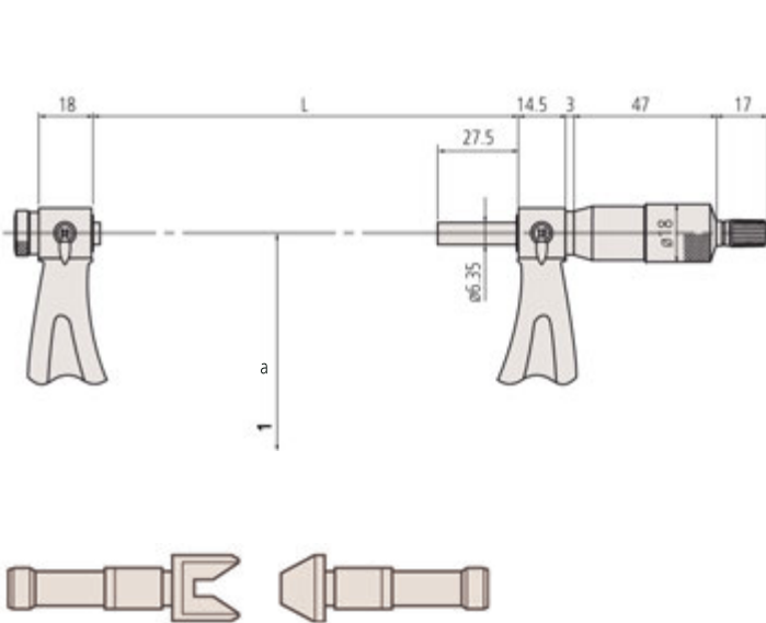
Aambeeld/spindel meetstift overeenkomend paar
