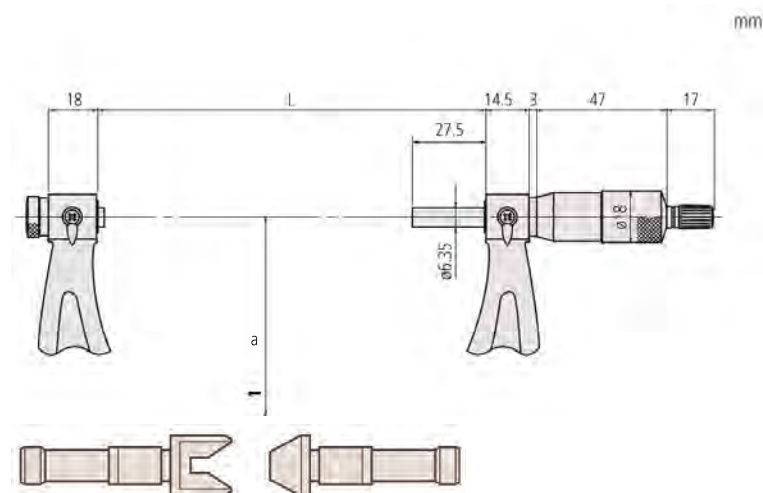
Aambeeld/spindel meetstift overeenkomend paar
