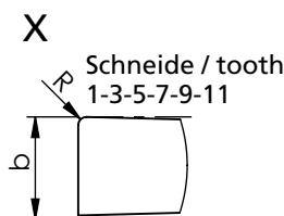
X1250.X kreuzverzahnt / staggered-toothed
