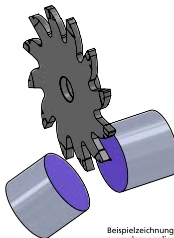
X1250.X kreuzverzahnt / staggered-toothed
